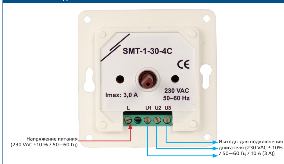
Рис. 1 Схема подключения
