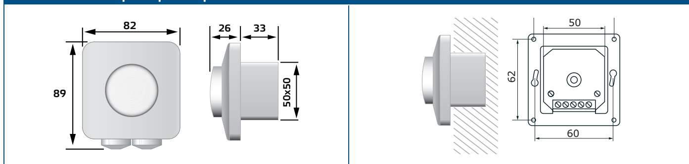
Рис. 2 Монтажные размеры - встроенный монтаж
